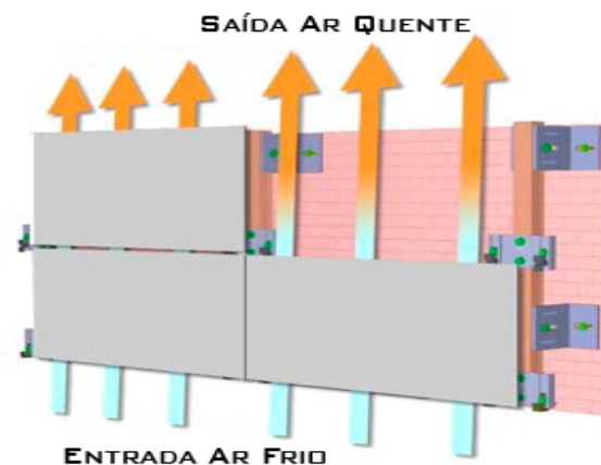
Figura 1. Ilustração Sistema de Fachada Ventilada (renovação do ar)
